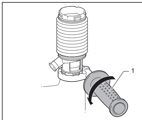
► 1. Empuñadura lateral
